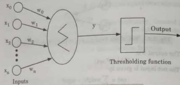
Fig. 2.10.1. Simple ADALINE network.
