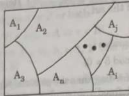
Fig. 3.9.1. Partition of set A.
