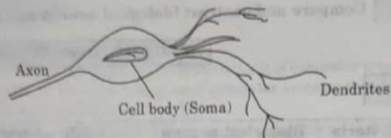
Fig. 1.7.1. Structure of neuron.
