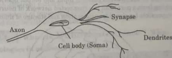
Fig. 1.1.1. Structure of neuron.
